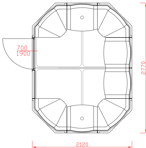
TYP 212/277 E
