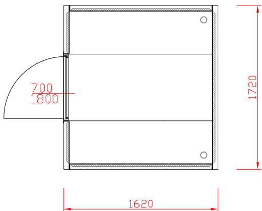
TYP 172/162
