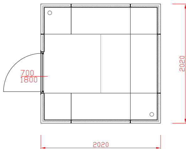
TYP 202/202
