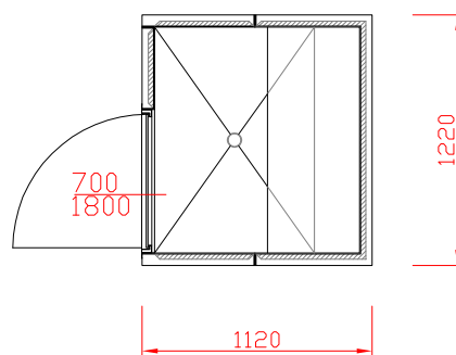
TYP 112/122
