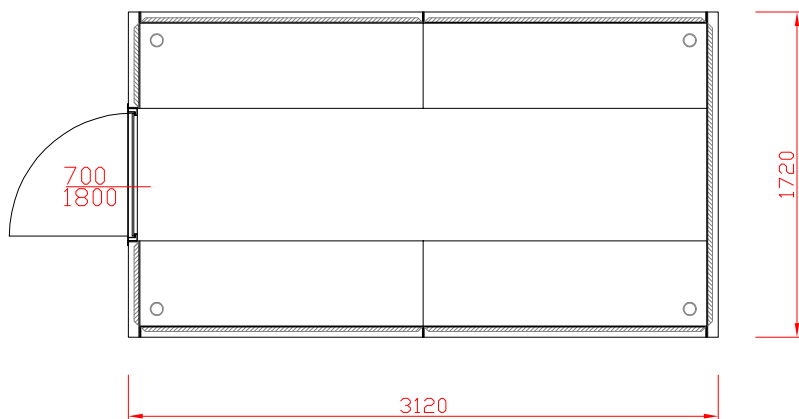
TYP 172/312
