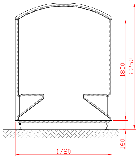
TYP 172
