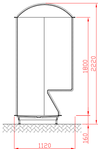
TYP 112/122
