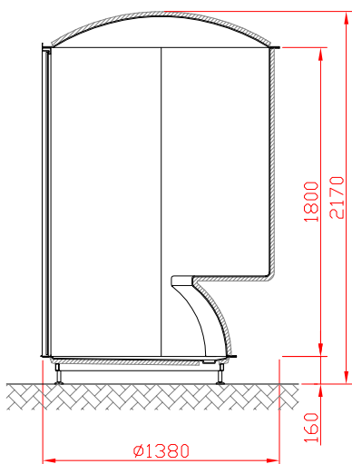
TYP 112/122
