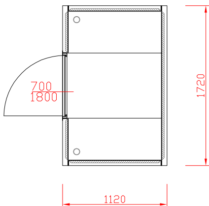
TYP 172/112
