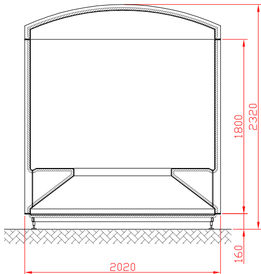
TYP 202
